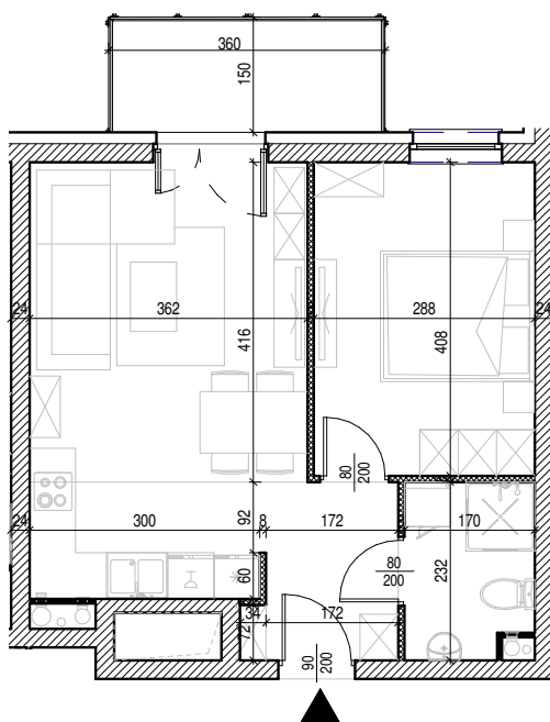
Rysunek architektoniczny
