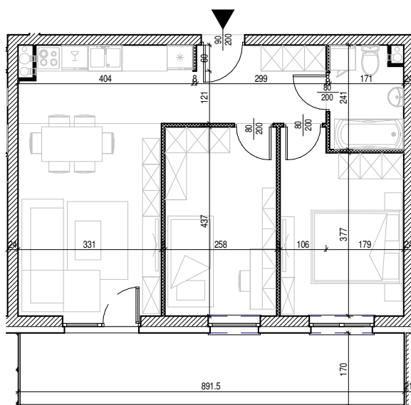
Rysunek architektoniczny
