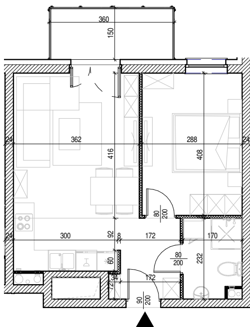
Rysunek architektoniczny
