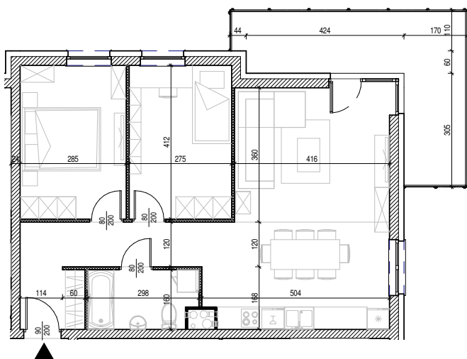
Rysunek architektoniczny
