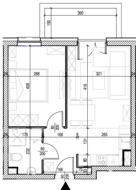
Rysunek architektoniczny
