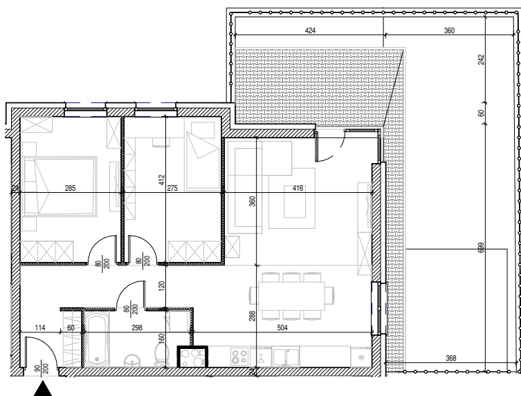
Rysunek architektoniczny
