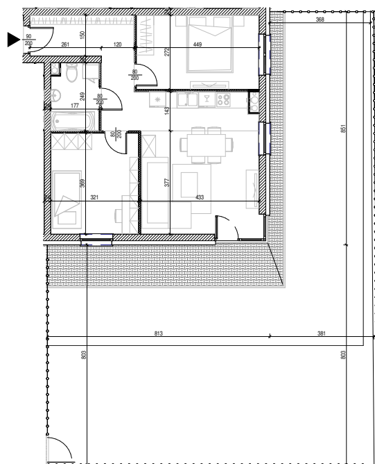
Rysunek architektoniczny
