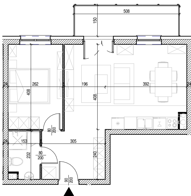
Rysunek architektoniczny
