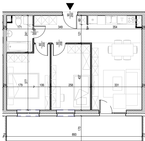
Rysunek architektoniczny
