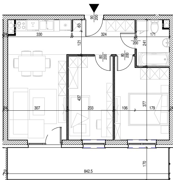
Rysunek architektoniczny
