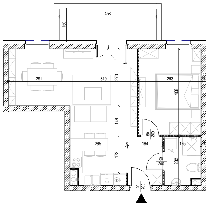
Rysunek architektoniczny
