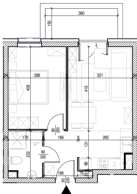
Rysunek architektoniczny
