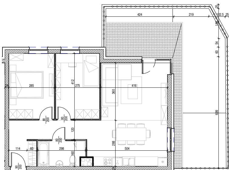
Rysunek architektoniczny
