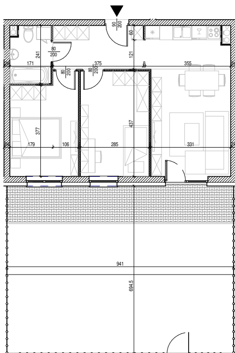
Rysunek architektoniczny
