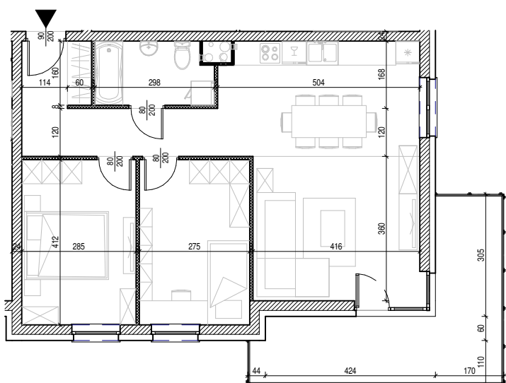
Rysunek architektoniczny
