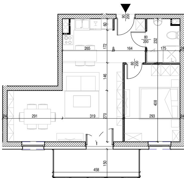
Rysunek architektoniczny
