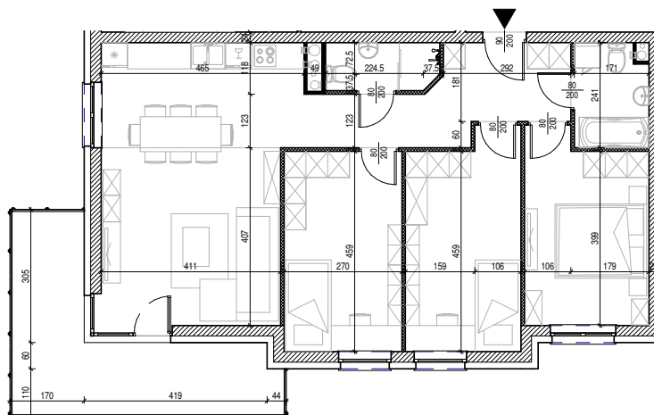
Rysunek architektoniczny
