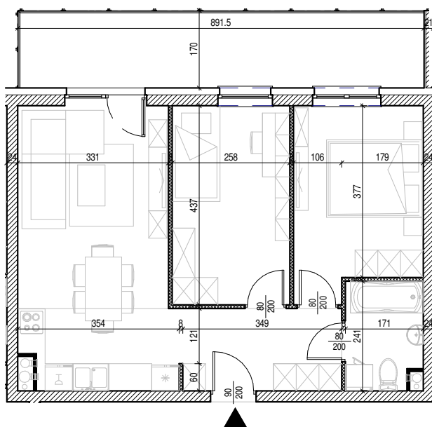
Rysunek architektoniczny
