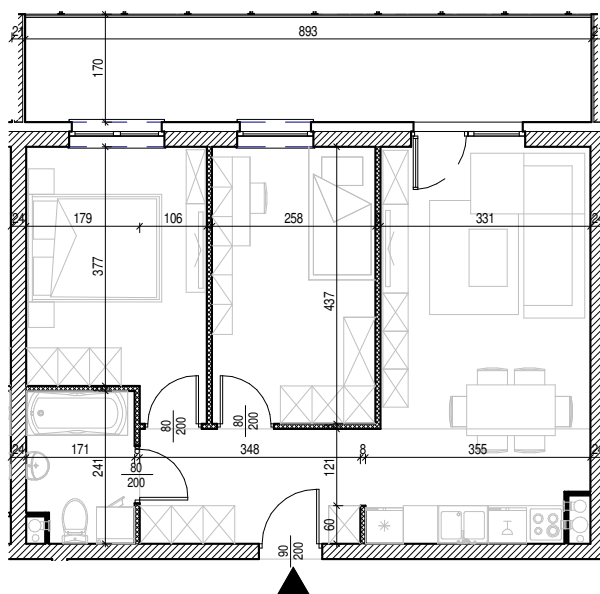
Rysunek architektoniczny
