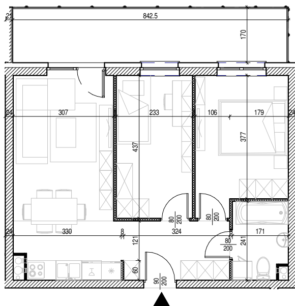
Rysunek architektoniczny
