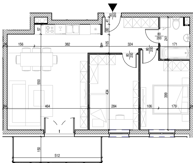
Rysunek architektoniczny
