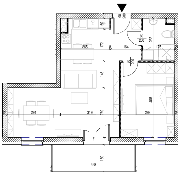
Rysunek architektoniczny
