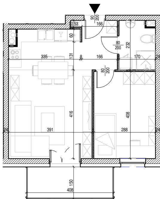
Rysunek architektoniczny
