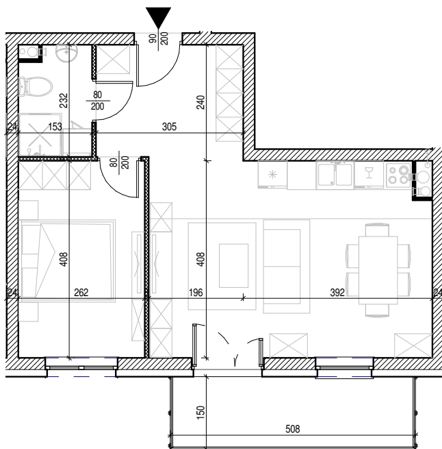
Rysunek architektoniczny
