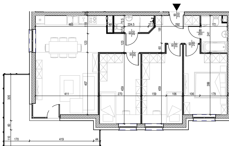
Rysunek architektoniczny
