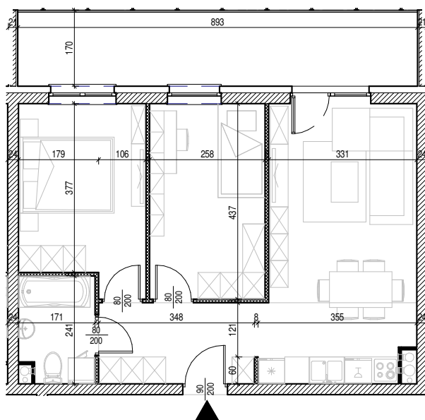
Rysunek architektoniczny
