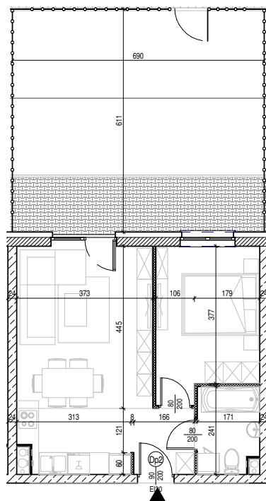
Rysunek architektoniczny
