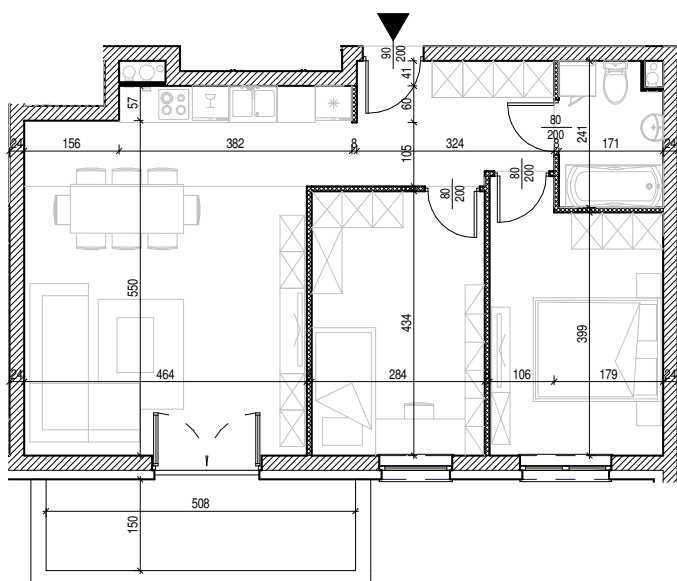
Rysunek architektoniczny
