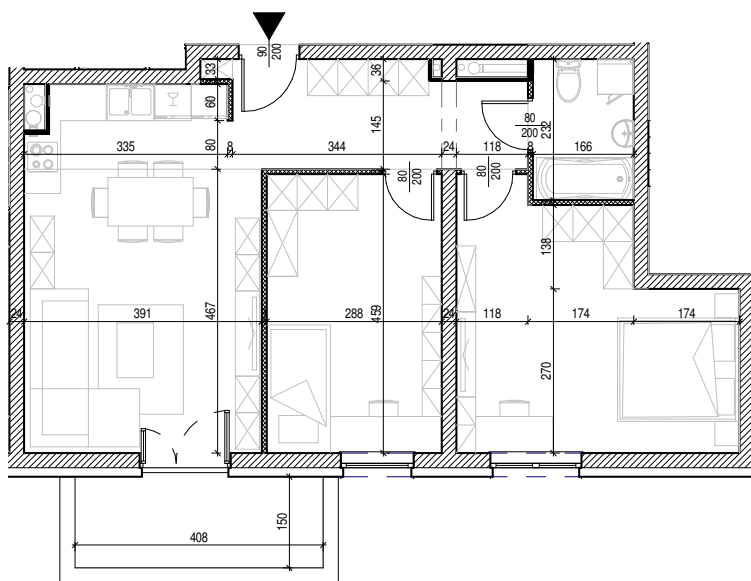
Rysunek architektoniczny
