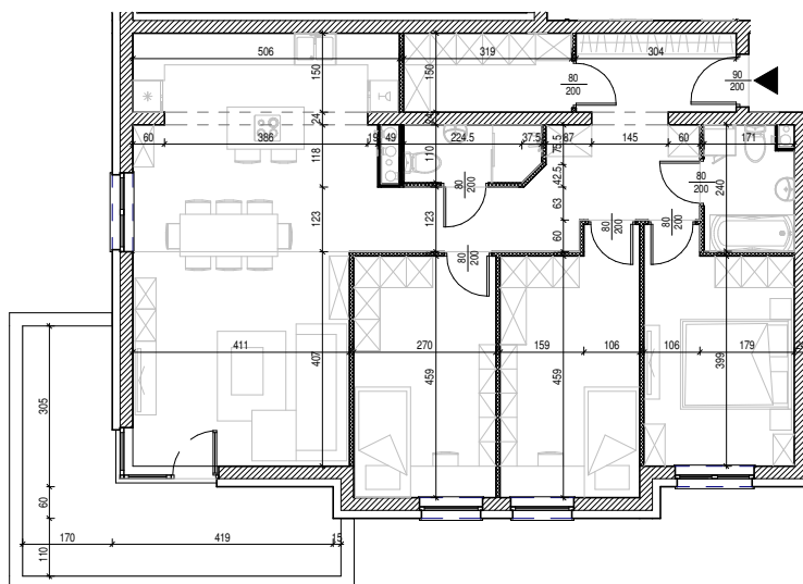
Rysunek architektoniczny
