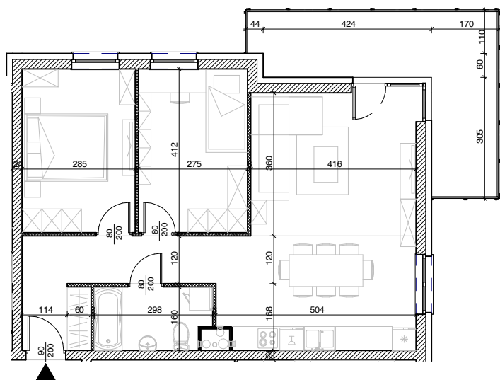
Rysunek architektoniczny
