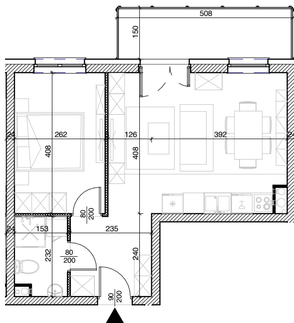
Rysunek architektoniczny
