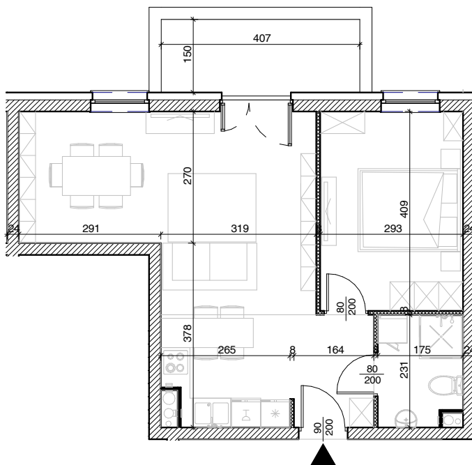
Rysunek architektoniczny
