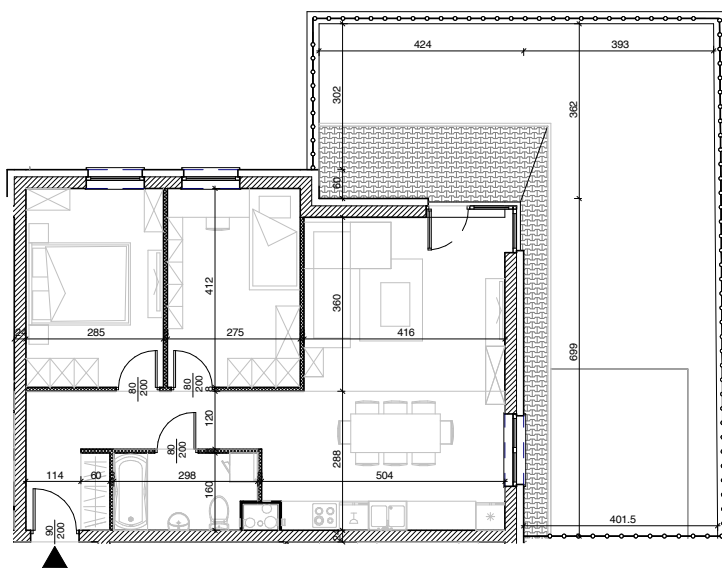
Rysunek architektoniczny
