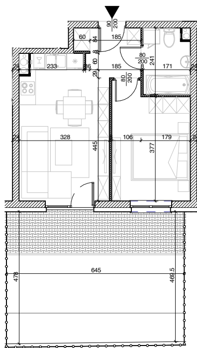
Rysunek architektoniczny
