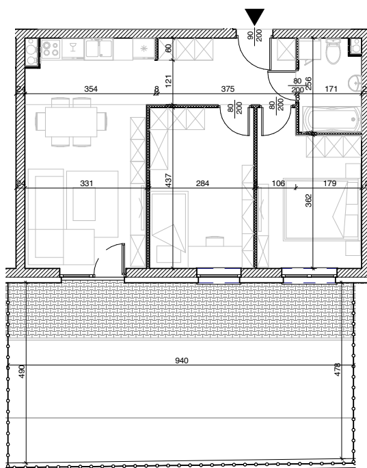
Rysunek architektoniczny
