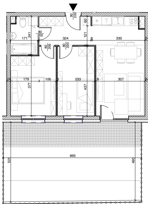
Rysunek architektoniczny
