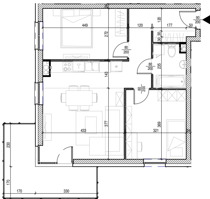
Rysunek architektoniczny
