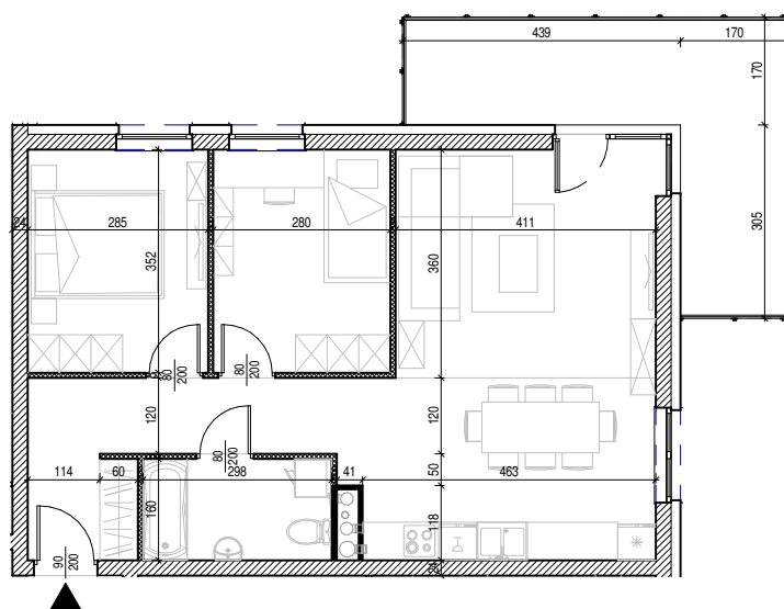
Rysunek architektoniczny
