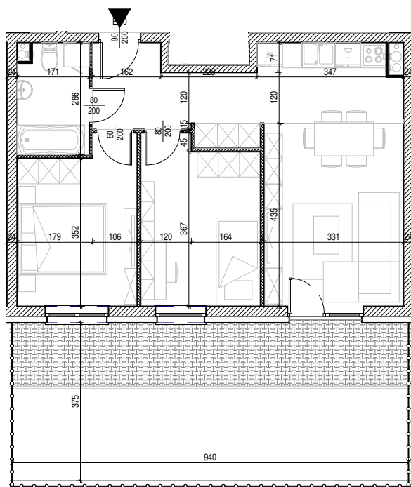
Rysunek architektoniczny
