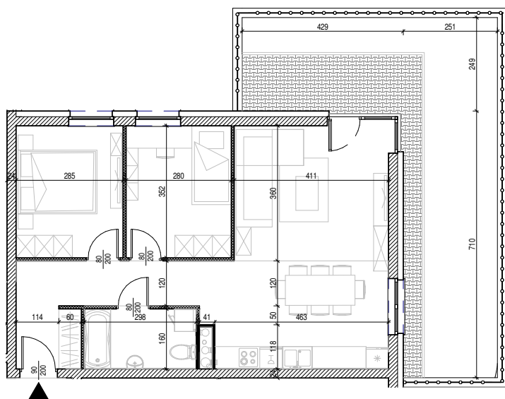
Rysunek architektoniczny
