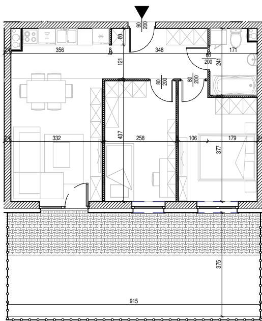
Rysunek architektoniczny
