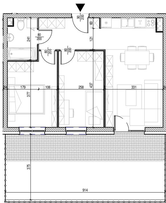
Rysunek architektoniczny
