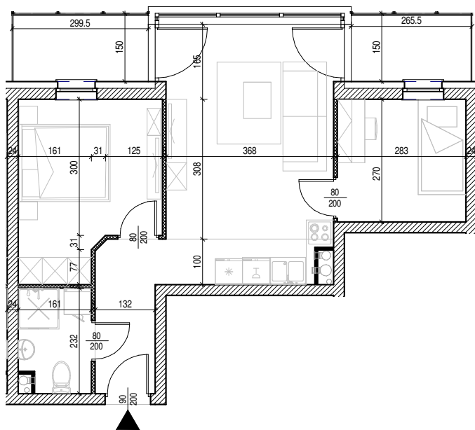
Rysunek architektoniczny
