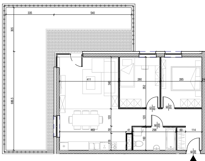
Rysunek architektoniczny
