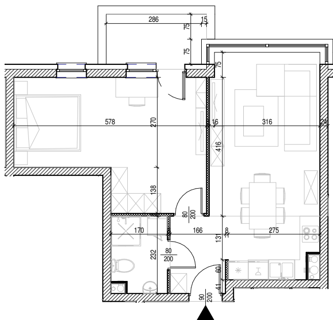
Rysunek architektoniczny
