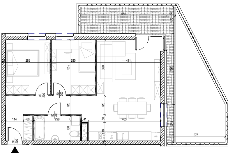
Rysunek architektoniczny
