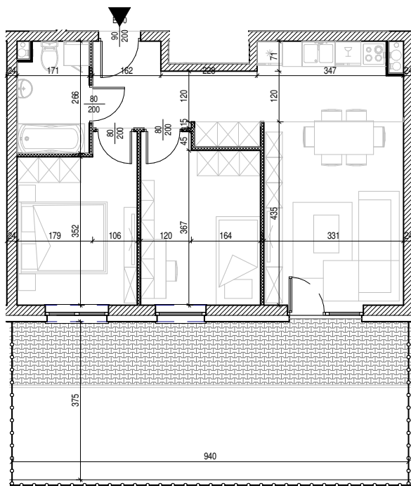
Rysunek architektoniczny
