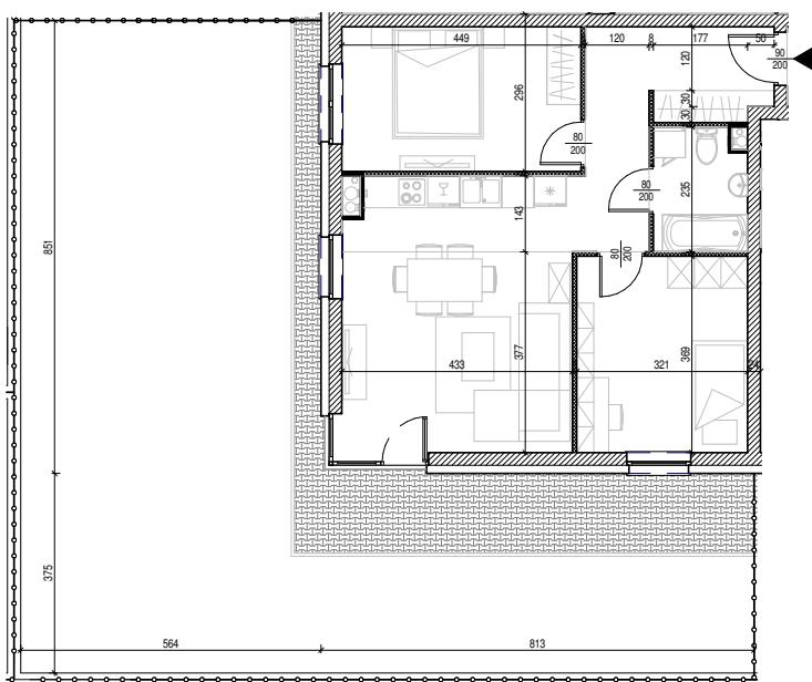
Rysunek architektoniczny
