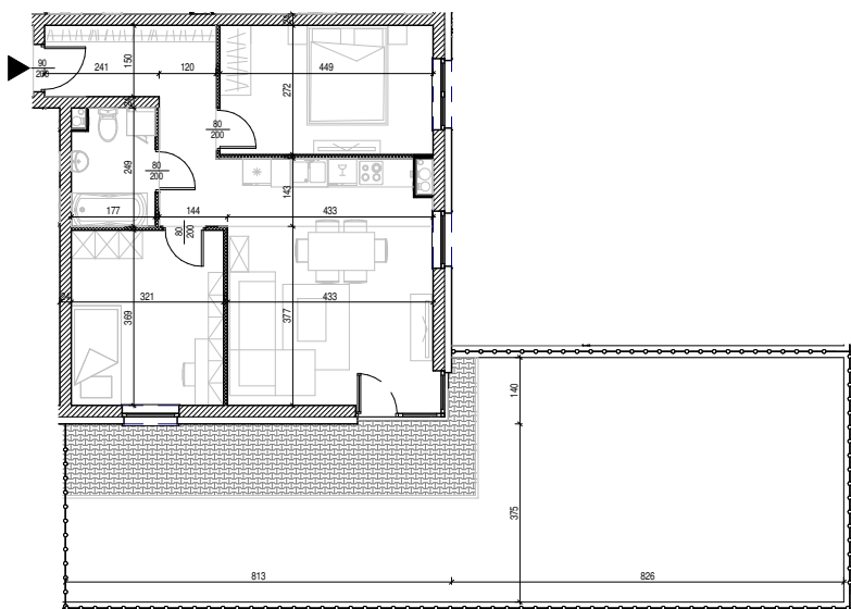
Rysunek architektoniczny
